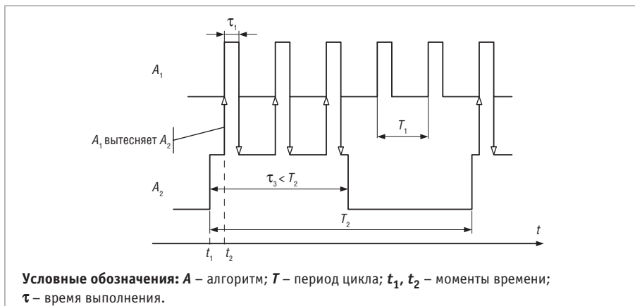
Рис. 7. Циклограмма исполнения алгоритмов разной срочности и длительности на контроллере с вытесняющей многозадачностью
